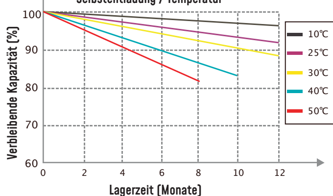
Selbstentladung / Temperatur
