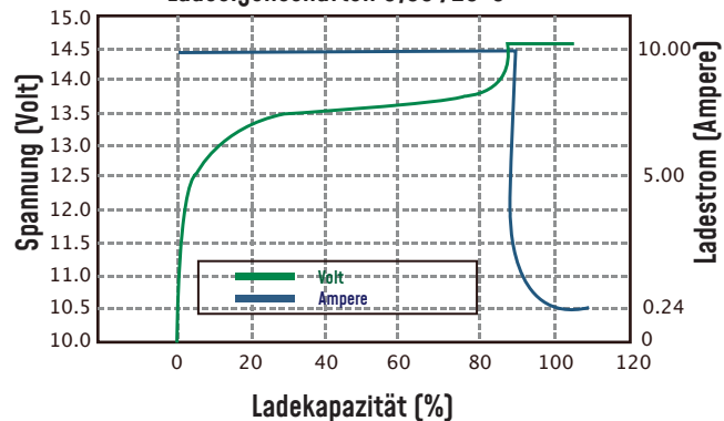
Ladeigenschaften 0,5C / 25°C
